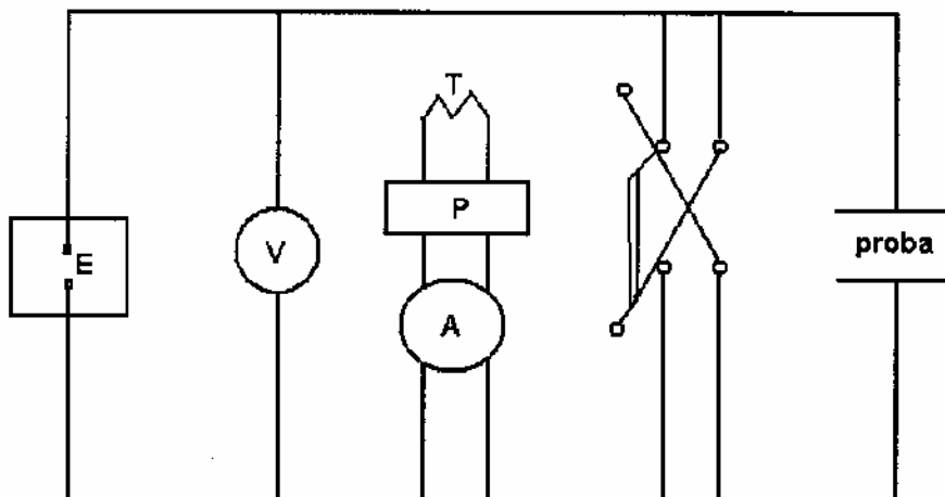
Schema instalației pentru studiul proprietăților electrice ale compuşilor revendicați E – sursă de curent; V - voltmetru electronic; A – miliampermetru pentru intensități mici; P – potențiomtru; T – termocuplu.
